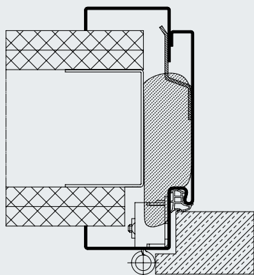
2-vrstvová zárubňa s ozdobným falcom a s prestavením hrúbky ostenia, falcované, upevnenie materiálovým stykom (2-zložková montážna pena) (do hmotnosti krídla dverí 50 kg)
