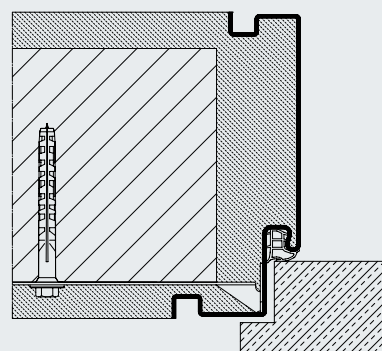
1-dielna zárubňa s omietkovou drážkou, falcovaná
