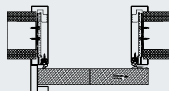
Zárubňa posuvných dverí posúvajúcich sa pred stenou, tesne zatvárajúce
