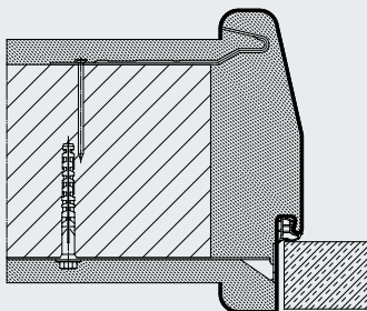
1-dielna zárubňa do muriva so zaobleným ostením, nefalcovaná
