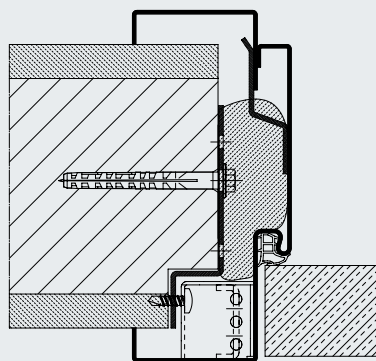
2-vrstvová zárubňa s ozdobným falcom a s prestavením hrúbky ostenia, nefalcované, skryto ležiaci záves, silové / materiálové spojenie (do hmotnosti krídla dverí 80 kg)
