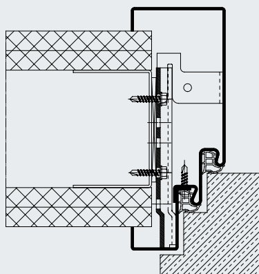
2-vrstvová zárubňa s dvojitém falcom, falcovaná
