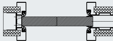
Zárubňa posuvných dverí posúvajúcich sa v stene, tesne zatvárajúce
