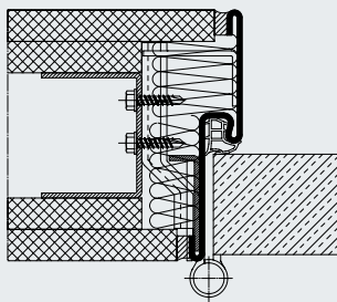
1-dielna zárubňa, nefalcovaná, pre montovanú stenu, systém závesov VN 2927 / 160 Compact Planum
