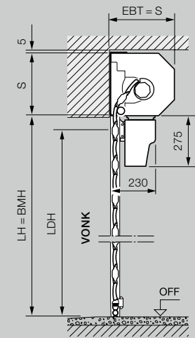
Rozsah veľkostí vnútorných a vonkajších rolovacích brán
