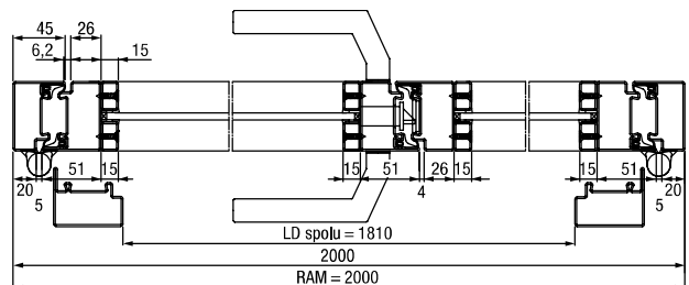
Horizontálny rez 2-krídlové oceľové dvere Loft
