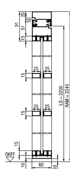
Vertikálny rez 1-krídlové oceľové dvere Loft
