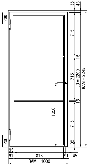
1-krídlové oceľové dvere Loft
