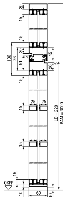
Vertikálny rez 2-krídlové oceľové dvere Loft s bočnými dielmi a nadsvetlíkom
