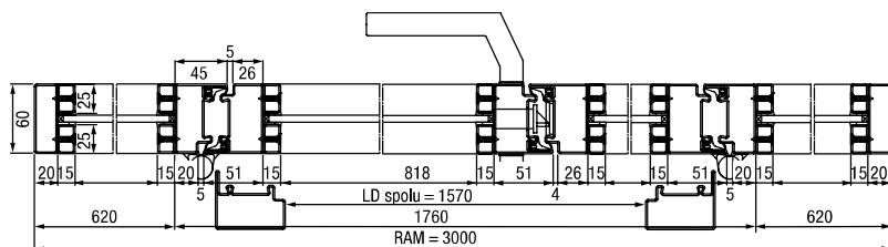
Horizontálny rez 2-krídlové oceľové dvere Loft s bočnými dielmi a nadsvetlíkom
