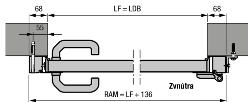
Vedľajšie dvere s hliníkovou blokovoú zárubňou typ profilu 1 Montáž za otvor
