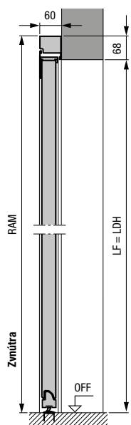
Vedľajšie dvere s hliníkovou blokovoú zárubňou typ profilu 2 Montáž za otvor
