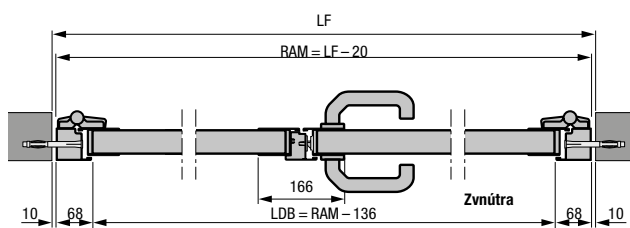
2-krídlové vedľajšie dvere s hliníkovou blokovoú zárubňou typ profilu 2 Montáž v otvore
