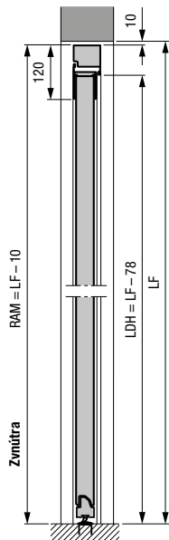
Vedľajšie dvere s hliníkovou blokovoú zárubňou typ profilu 2 Montáž v otvore
