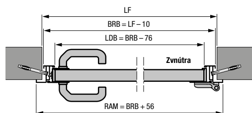
Vedľajšie dvere s hliníkovou rohovoú zárubňou typ profilu 1 alebo 2 Vnútroň doraz
