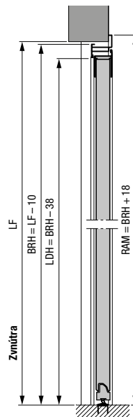
Vedľajšie dvere s hliníkovou rohovoú zárubňou typ profilu 2 Vonkajší doraz
