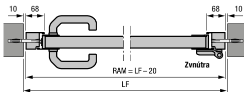
Vedľajšie dvere s hliníkovou blokovoú zárubňou typ profilu 2 Montáž v otvore
