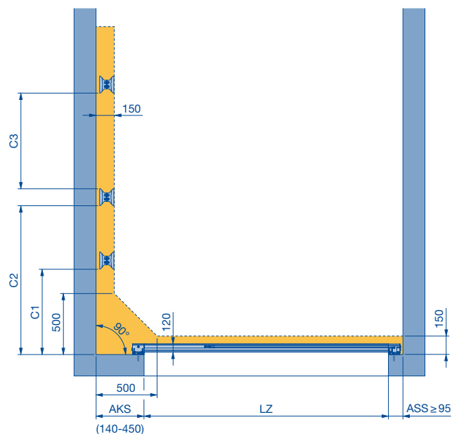
Rez podlahovej koľajnice
