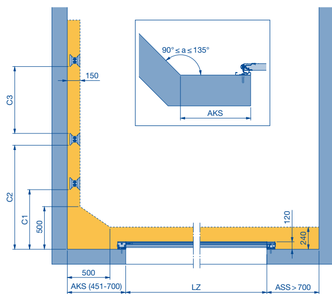
Rez podlahovej koľajnice
