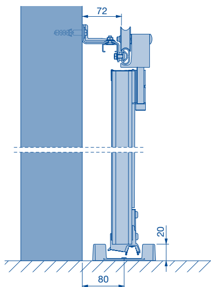
Bočná stena – kovanie DS horné ukončenie
