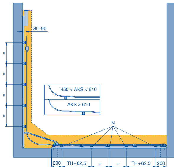
Rez vodiacej koľajnice
