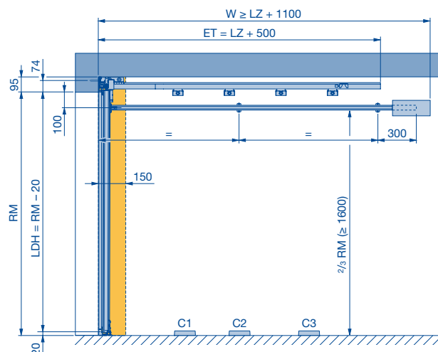
Rez vodiacej koľajnice
