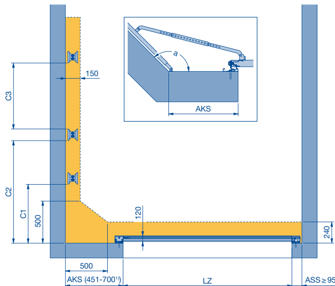
Rez podlahovej koľajnice
