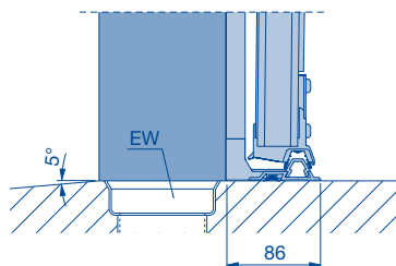
Podlahové ukončenia s odvodnením (EW)
