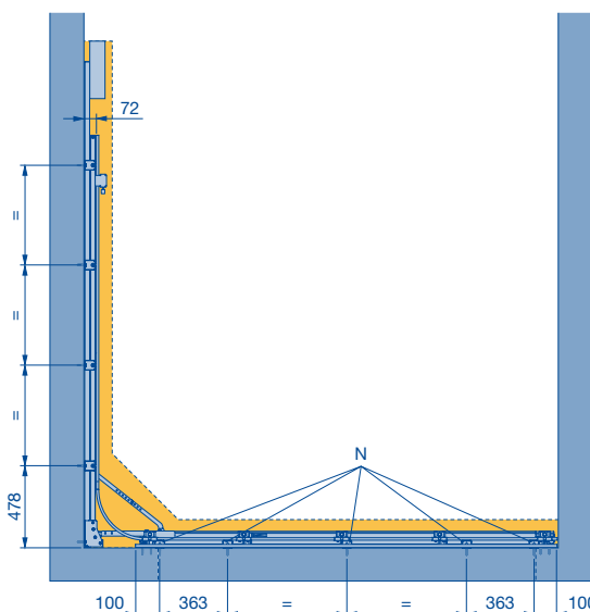
Rez vodiacej koľajnice
