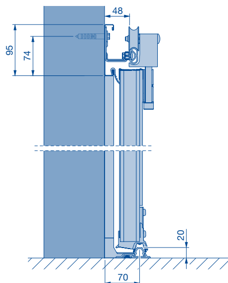
Predná stena horné ukončenie
